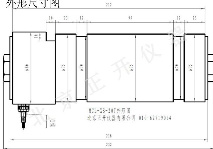
外形尺寸图
